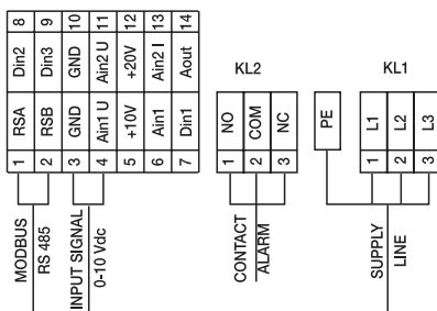
Collegamenti elettrici Electrical connections KL3
