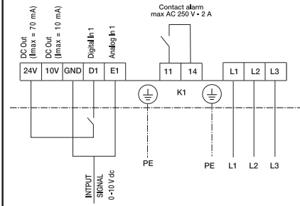
Versione OPTIONAL (Modbus) OPTIONAL version (Modbus)
