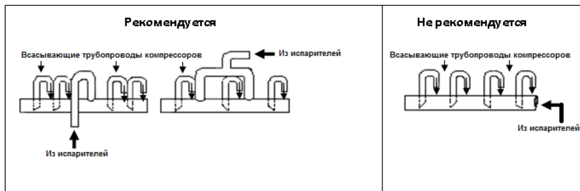
Рис. 6: Коллектор всасывания - рекомендации
