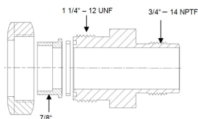
Рис 5: Адаптер для смотрового стекла
