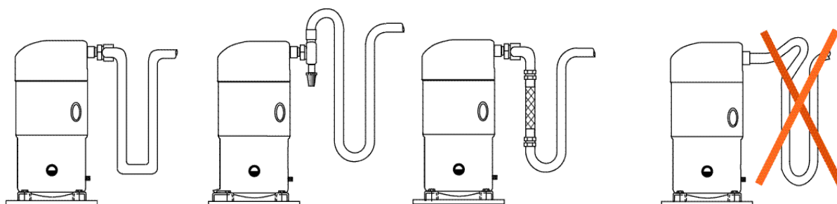
Рис. 7: Рекомендации по трубной обвязке
