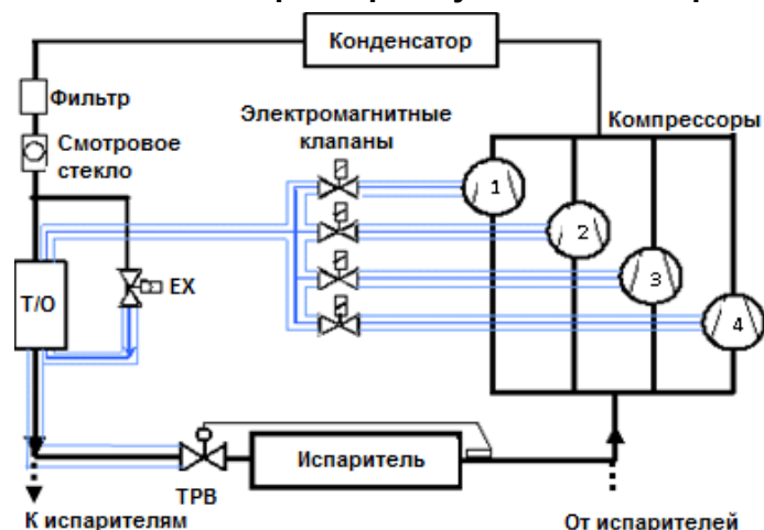
Рис. 8: Многокомпрессорная установка с общим экономайзером
