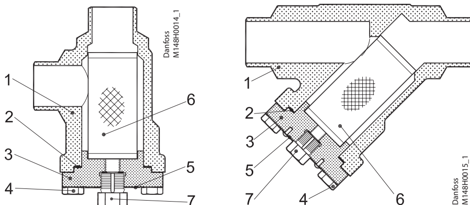
FIA 15-40 (1/2 - 1 1/2 дюйма)
