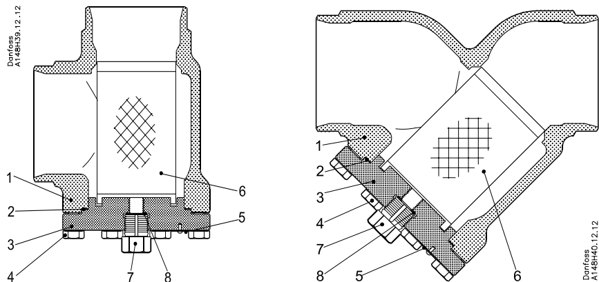
FIA 50 - 200 (2 - 8)
